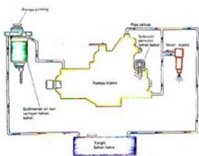
Gambar 47. Sistem bahan bakar engine disel dengan pompa rotary
