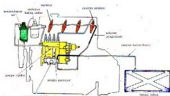
Gambar 46. Sistem bahan bakar engine disel dengan Pompa In-line
